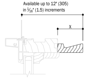
G Extension Jamb
